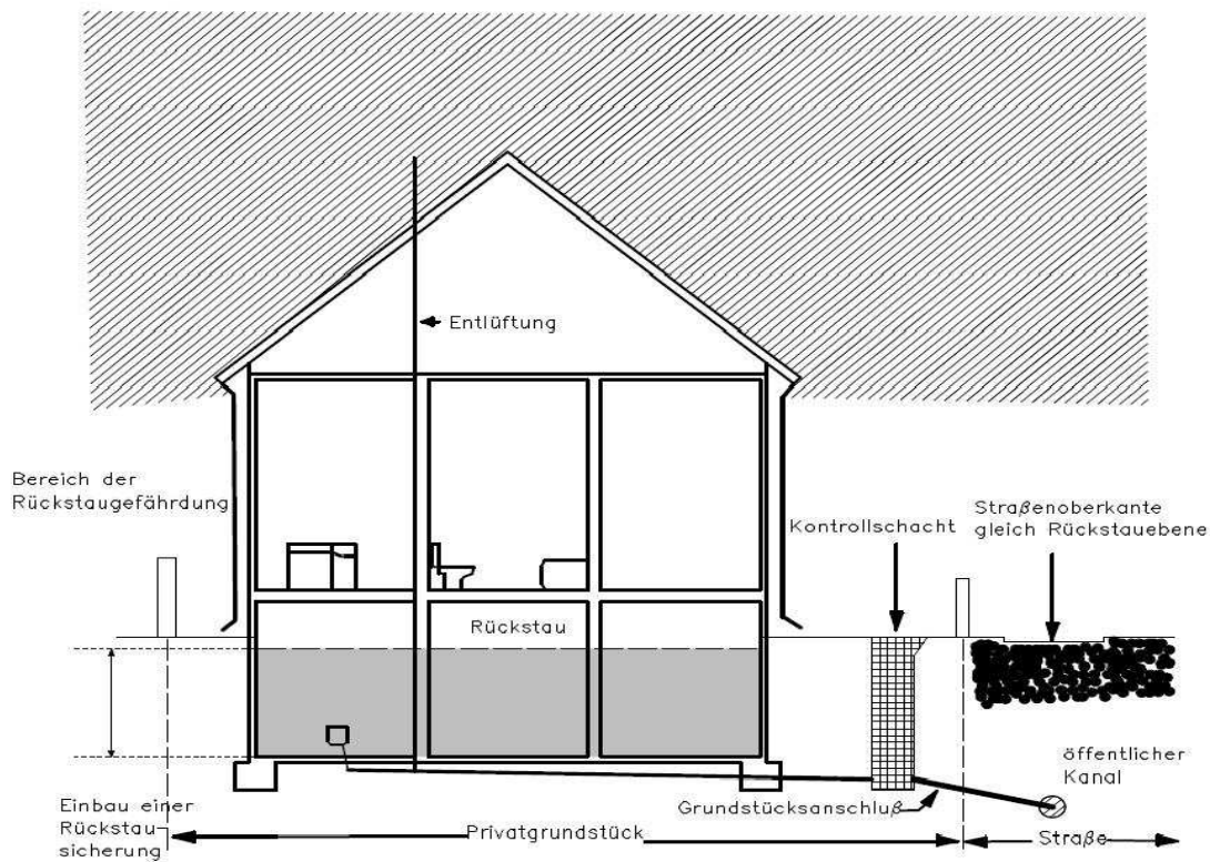
Skizze "Rückstauoberkante"
